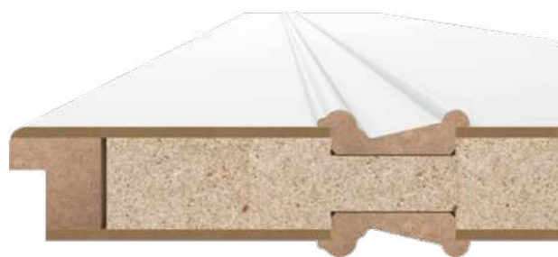
Schnitt Cottage, Standardeinlage VSP
