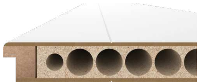
Standardeinlage V-Nut Fräsung
