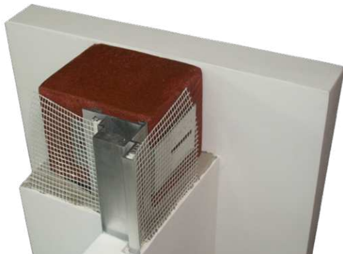
Detailansicht TCS
