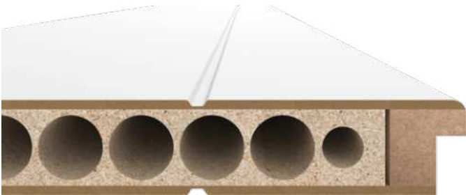
Schnitt Luana, Standardeinlage RSP
