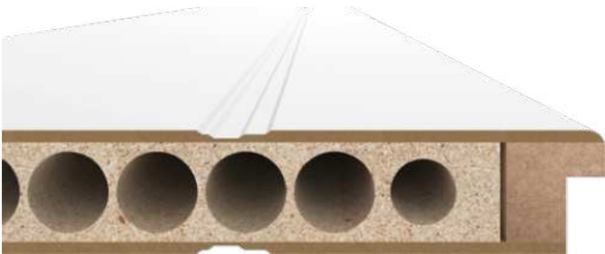
Schnitt Chello, Standardeinlage RSP
