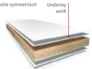
MW Aufbau (Bsp. MW03) Aufbau Oberseite und Unterseite symmetrisch
